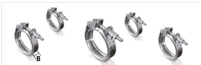
V-Band Ersatzschelle mit Schnellverschluß (passend für V-Band Kupplungsstück)
